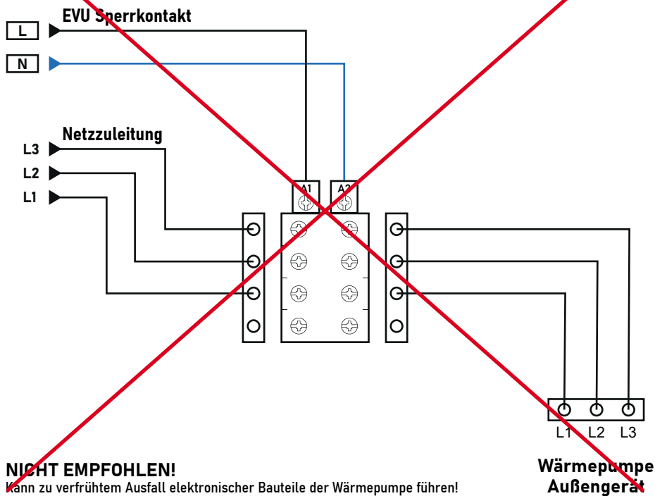
Abb. 16: Anschluss EVU-Sperre
