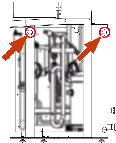
Abb. 13: Gerät auf Sockel montieren
