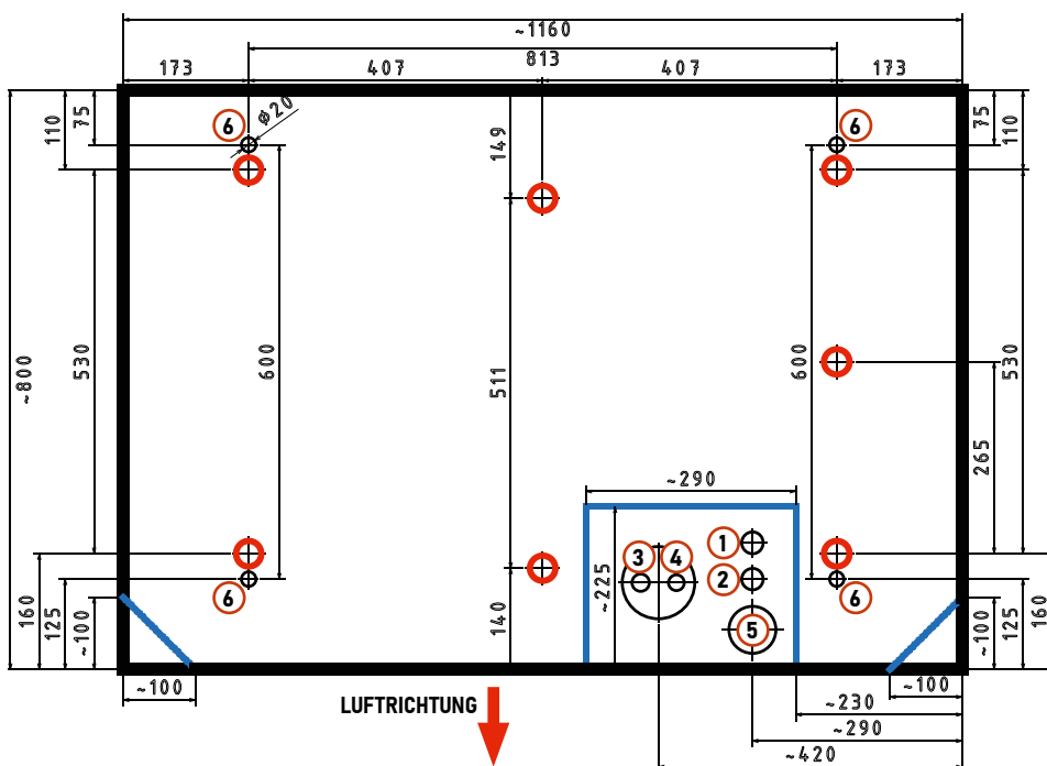
Abb. 12: Sockelplan EU20L
