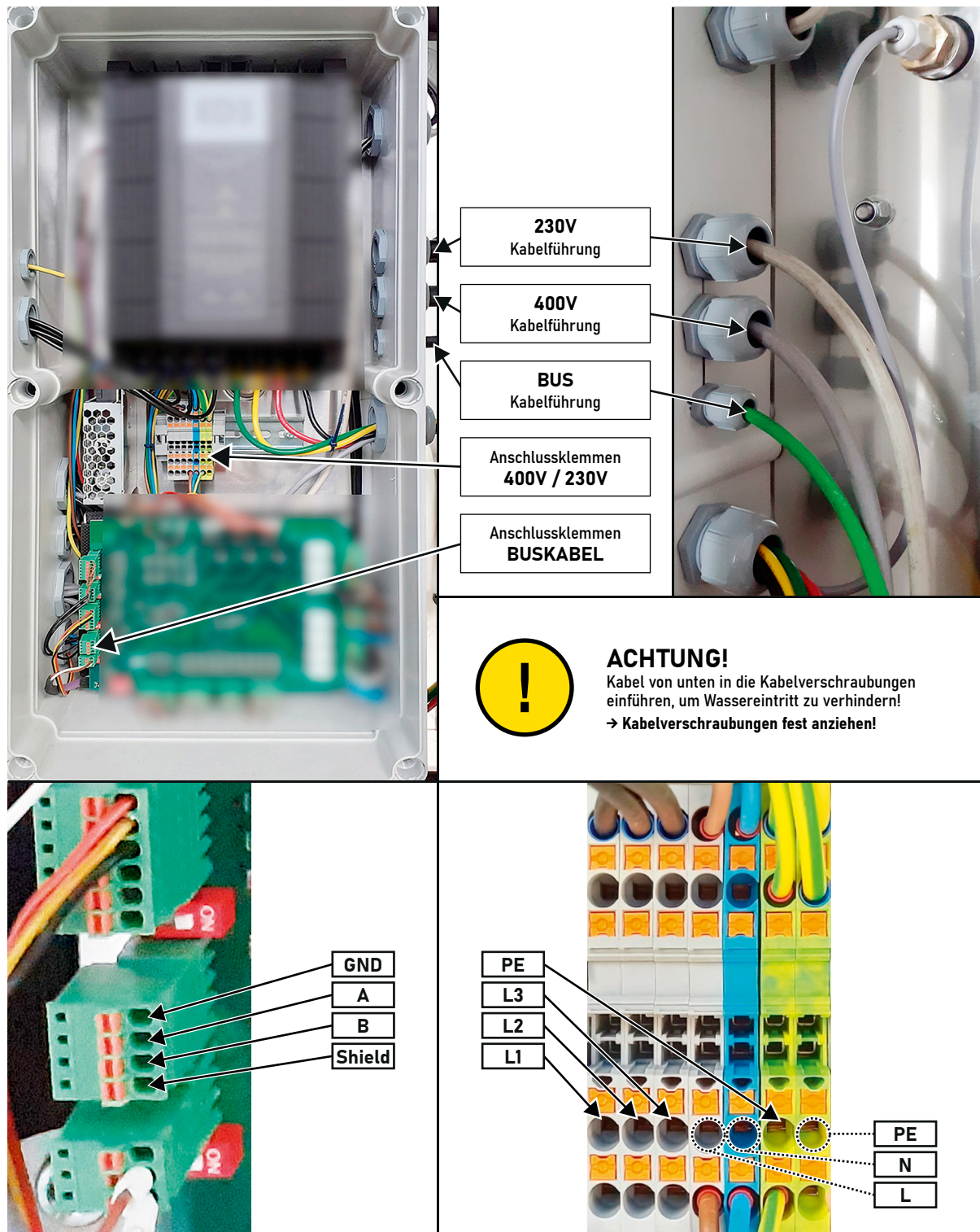
Abb. 17: Elektrischer Anschluss Außeneinheit
