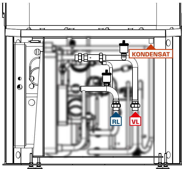
Abb. 14: Hydraulik anschließen
