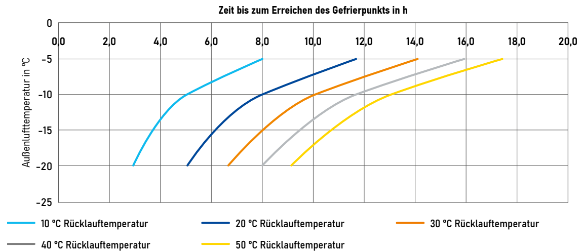
Abb. 22: Zeitdauer bis zum Erreichen des Gefrierpunkts in den wasserführenden Bauteilen der Wärmepumpe
