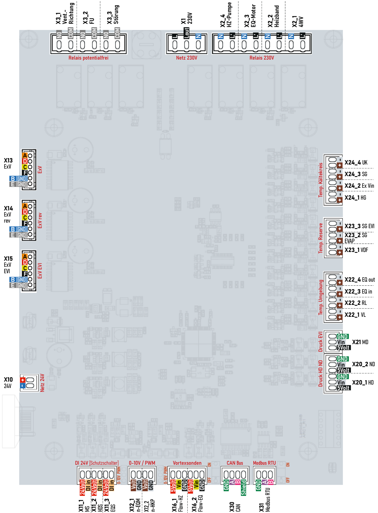
Abb. 18: Anschlussklemmen ARC Kältekreisregler
