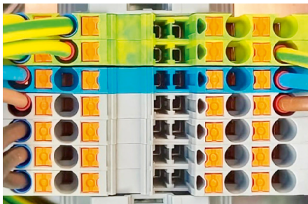
Abb. 15: Übersicht Verkabelung
