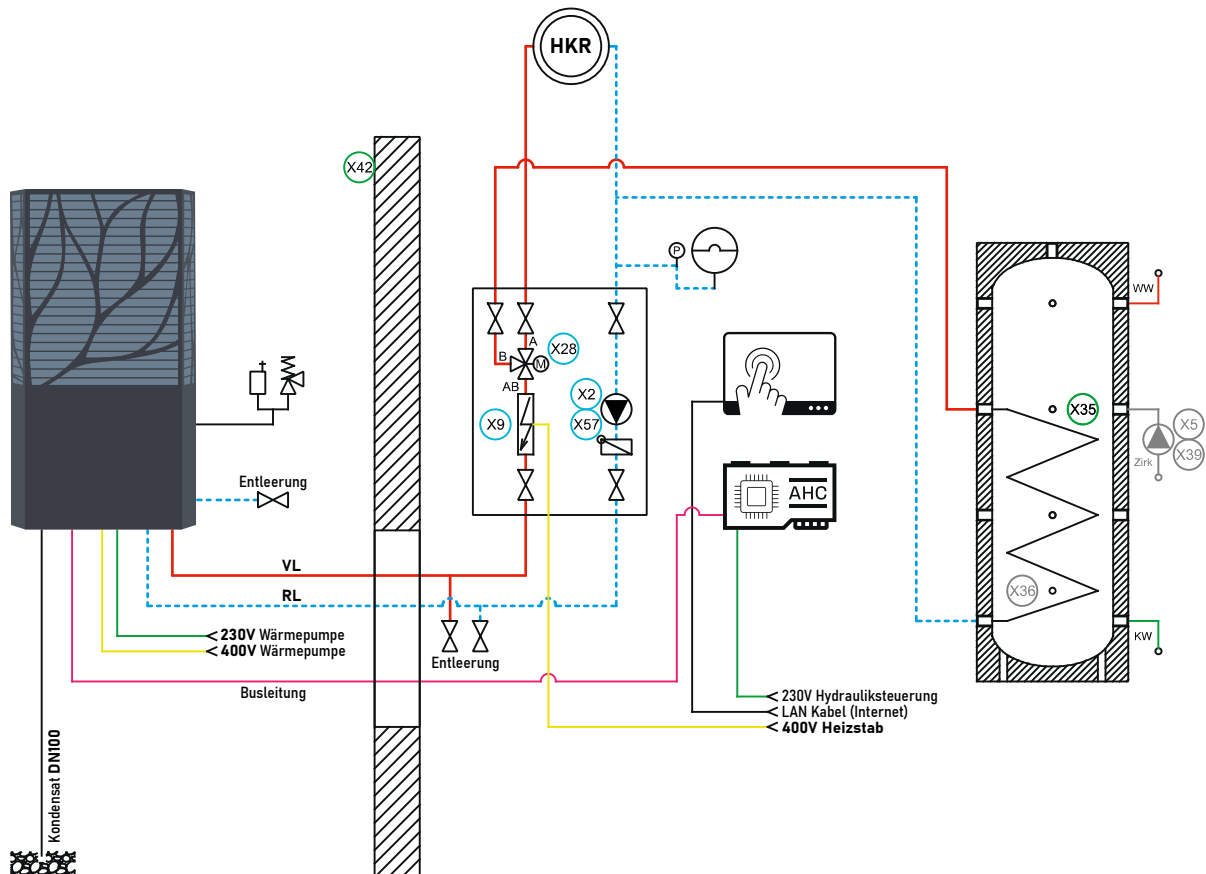
Abb. 1: Prinzipschema 111_000
