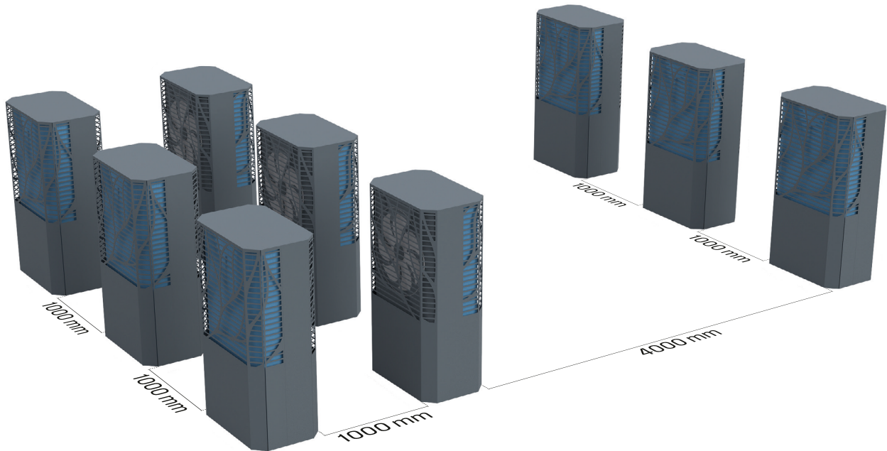
Abb. 10: Mindestabstand bei Kaskadenaufstellung
