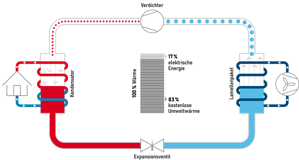
Abb. 2: Funktionsprinzip
