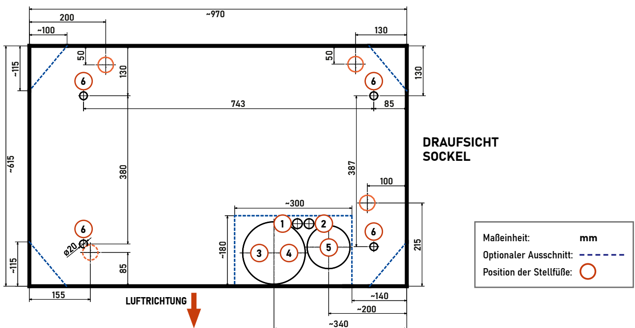
Abb. 11: Sockelplan Prinzipschema EU10L, EU13L und EU15L
